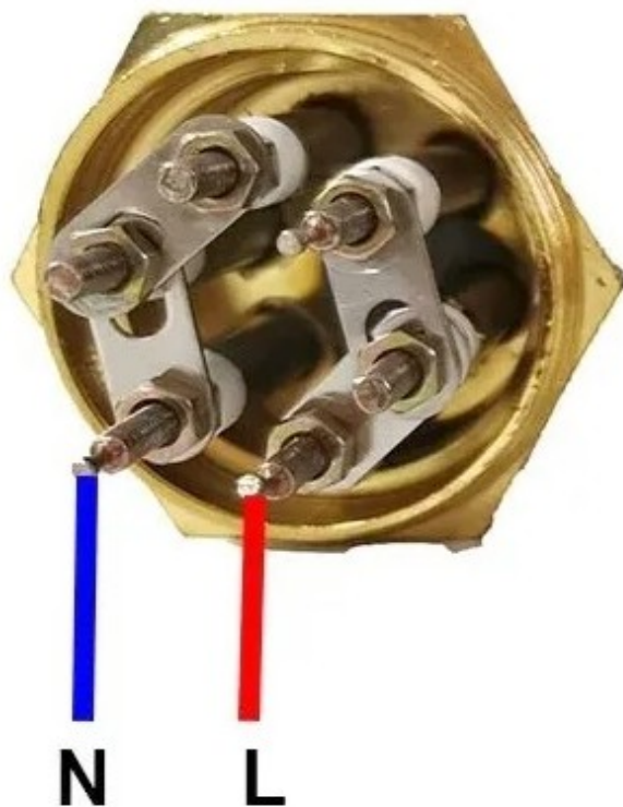
CONEXION 230v
